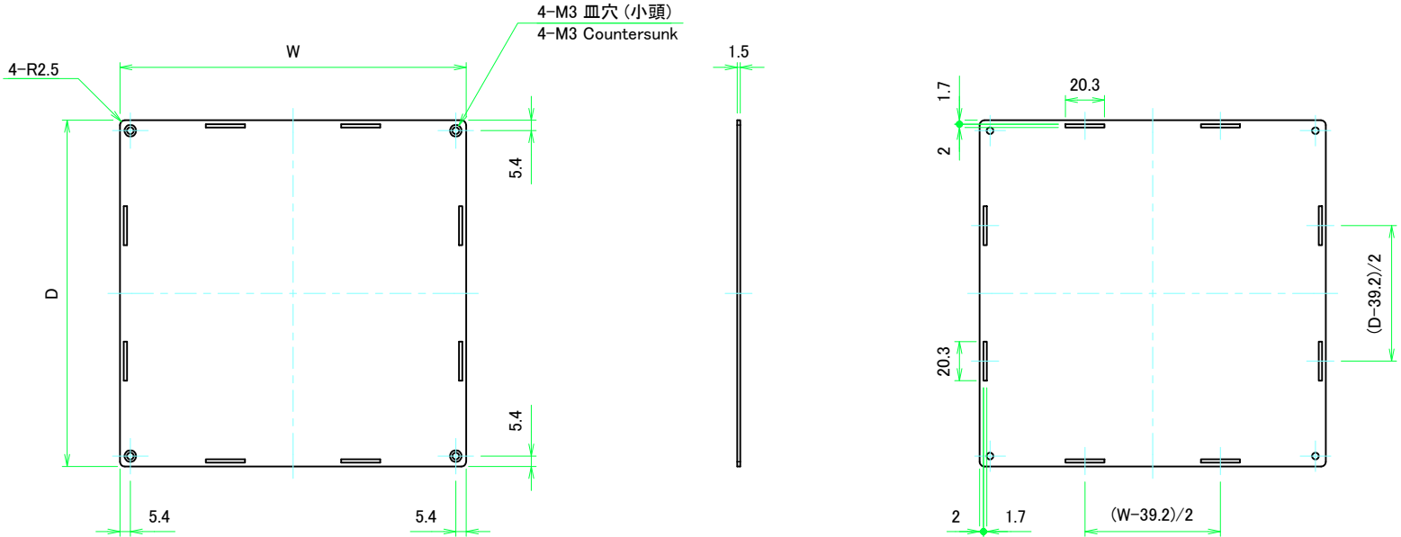
上カバー裏面 / Top cover Backside
